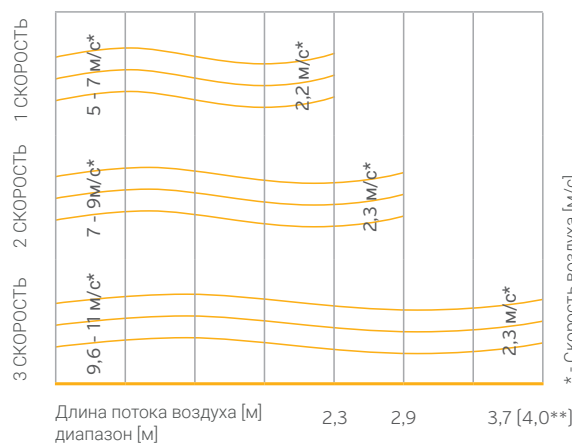
Длина горизонтальной струи воздуха (при вертикальном монтаже)
